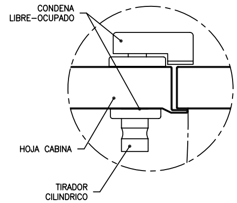
DETALLE SOLAPE HOJA
