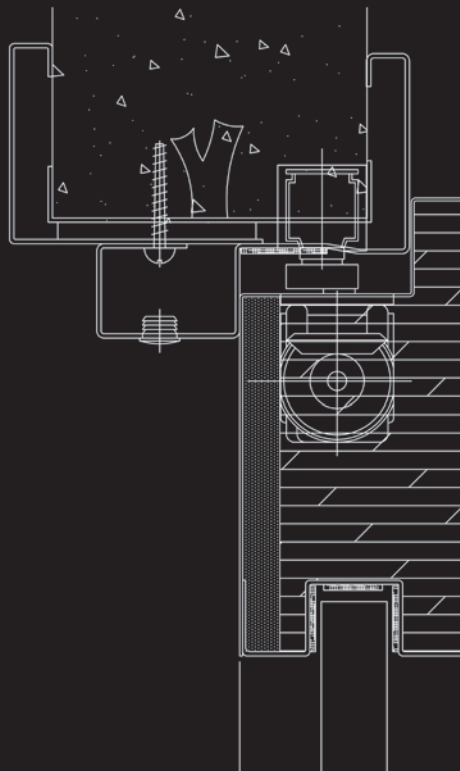
PUERTA VIDRIADA CORTAFUEGOS MUELLE OCULTO
