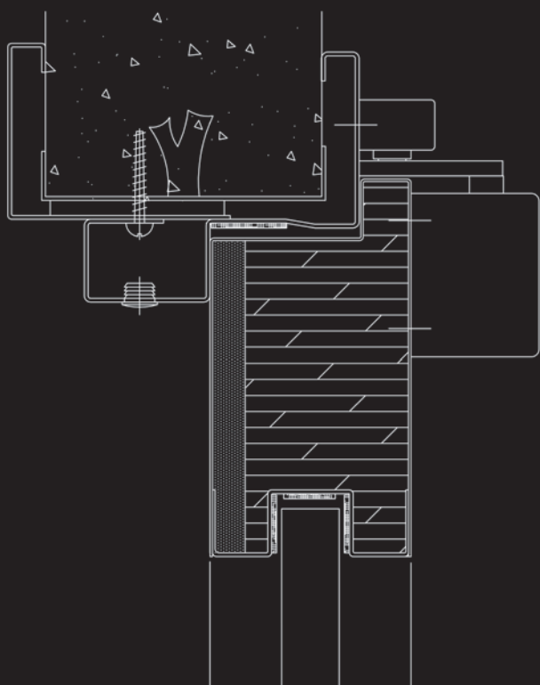
PUERTA VIDRIADA CORTAFUEGOS MUELLE AÉREO
